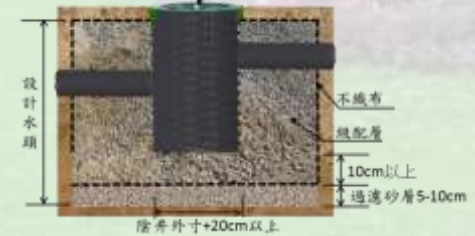
圖3-24 雨水滲透陰井組合設置示意圖
