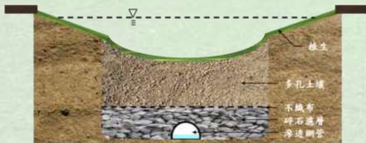
圖3-3 雨水滲透草溝示意圖
