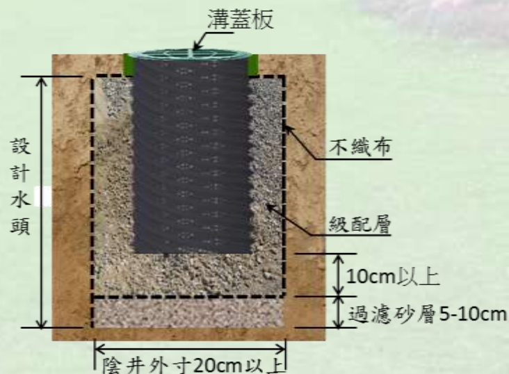
圖3-26 雨水滲透側溝斷面示意圖
