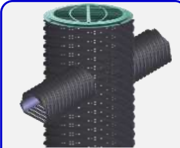
RCM-滲透井基地保水系統 Rainwater Conservation Module
