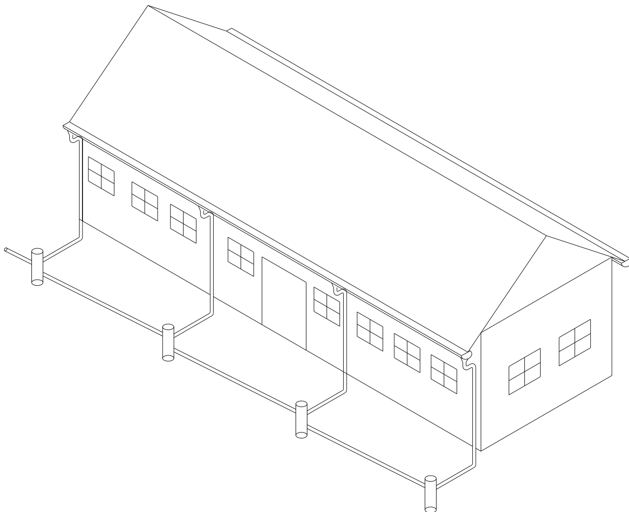
圖三 屋頂排水範例屋設計示意圖一
