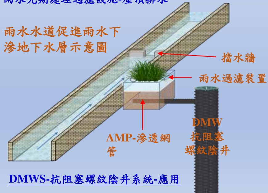
雨水先期處理過濾設施-屋頂排水
