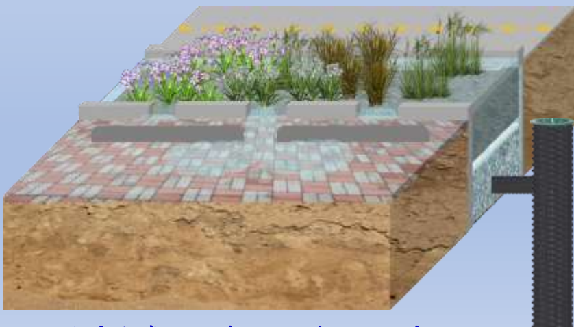
雨水先期處理過濾設施-道路安全島
